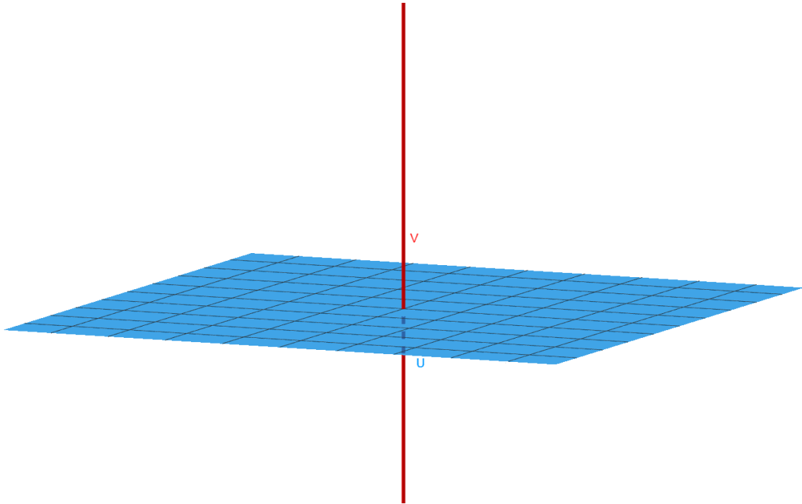
Figura 7.3: Ortogonalidade em \mathbb{R}^3 (arquivo pessoal)
