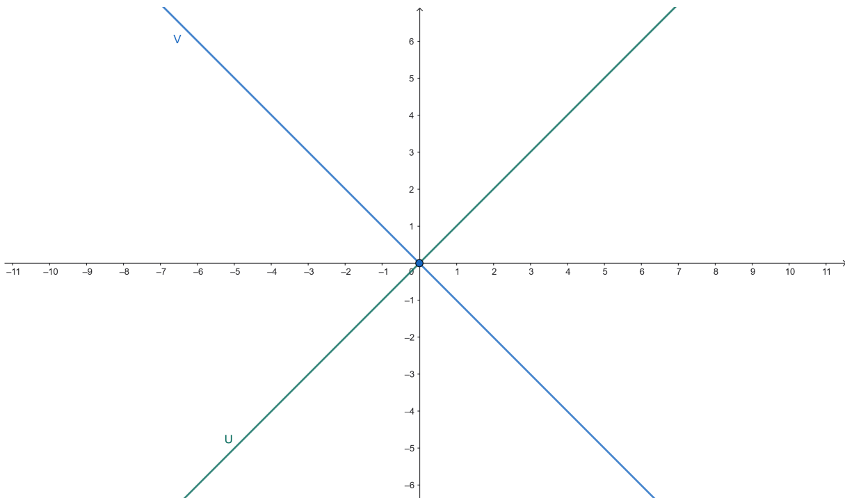
Figura 7.2: Ortogonalidade em \mathbb{R}^2 (arquivo pessoal)
